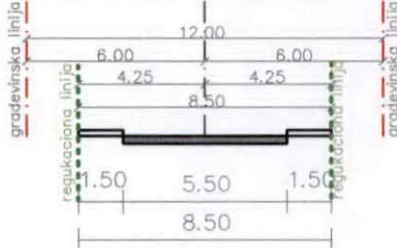
presjek D-D
