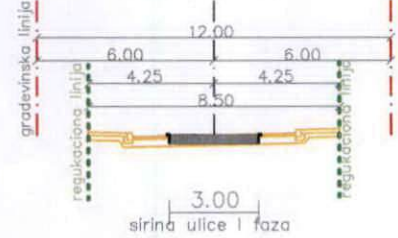
presjek P-P
